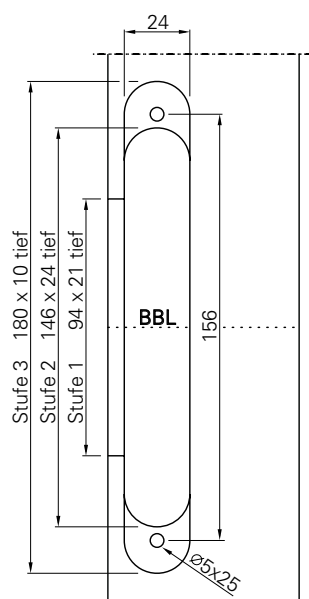
铣切图示
