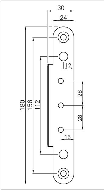
装饰外盖尺寸 OBX-3097
