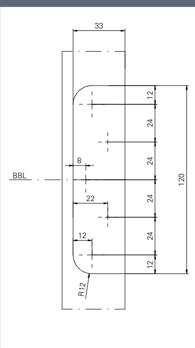
铣切图示
