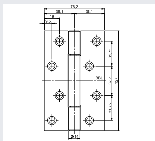
OBN-14 5030 Z 方角
