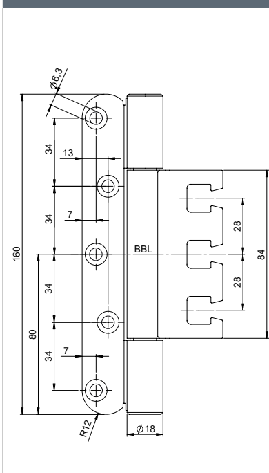
产品尺寸图
