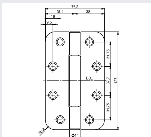
OBN-14 5030 C 圆角
