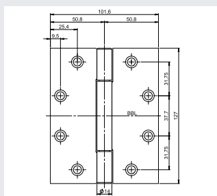
OBN-14 5040 C 方角
