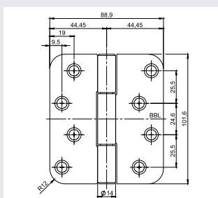
OBN-14 4035 Z 圆角
