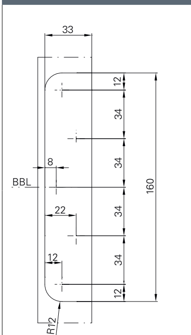
铣切图示
