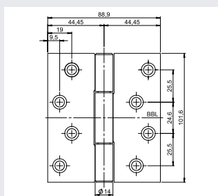
OBN-14 4035 Z 方角
