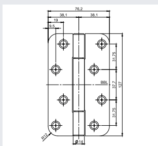
OBN-14 5030 Z 圆角
