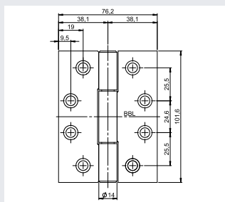
OBN-14 4030 C 方角
