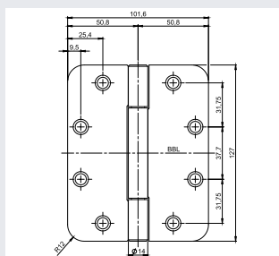
OBN-14 5040 C 圆角
