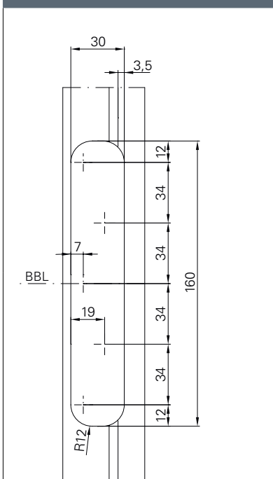
铣切图示
