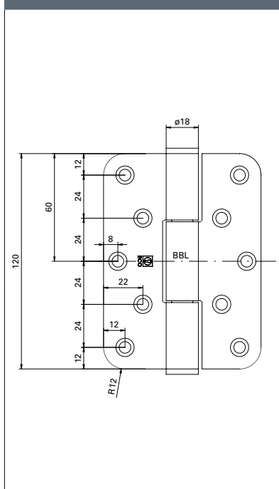
产品尺寸图
