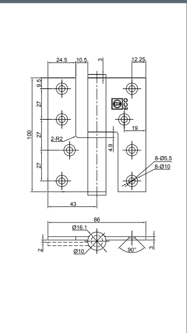
产品尺寸右手门图: 4" * 3.5" * 3
