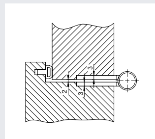
安装示意图
