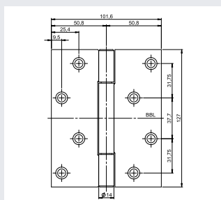
OBN-14 5040 Z 方角
