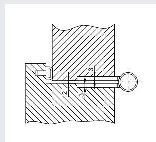
安装示意图
