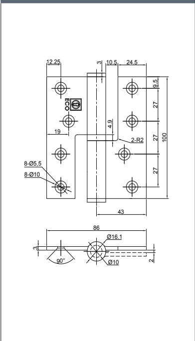
产品尺寸左手门图: 4" * 3.5" * 3
