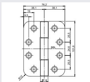
OBN-14 4030 C 圆角
