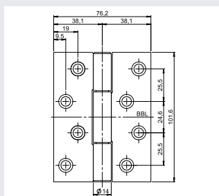
OBN-14 4030 Z 方角
