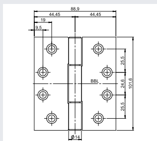
OBN-14 4035 C 方角
