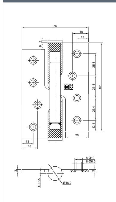
产品尺寸右手门图:
