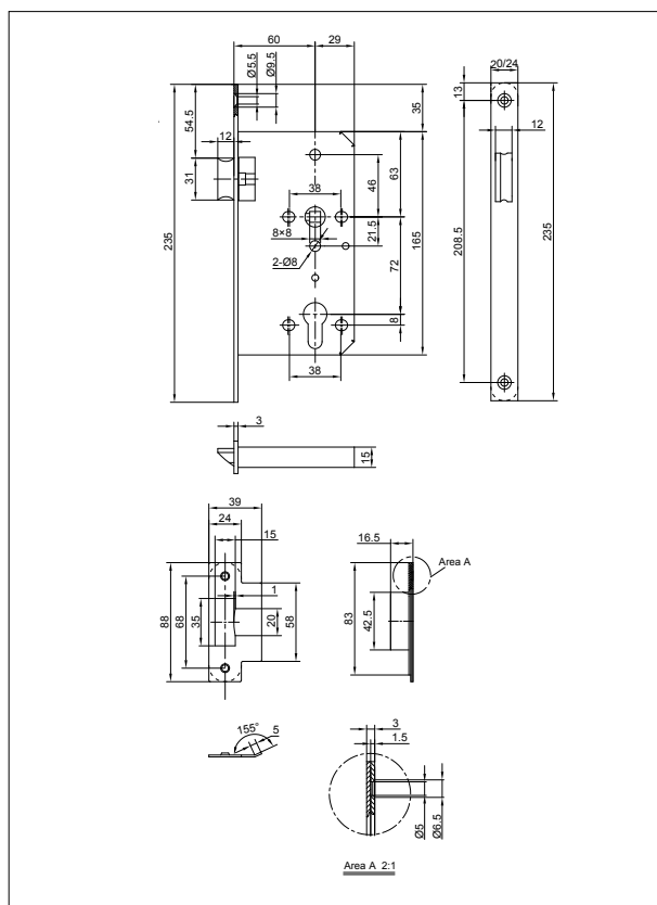
尺寸图: GBS 31 F UR 锋舌锁
