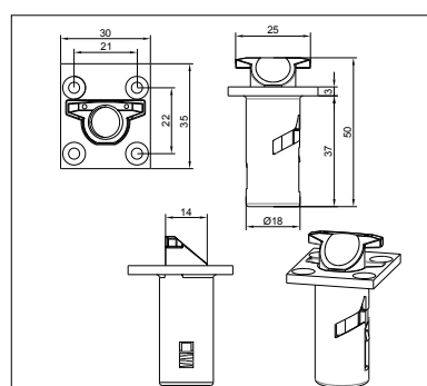
尺寸：门扇上置式调整锁
