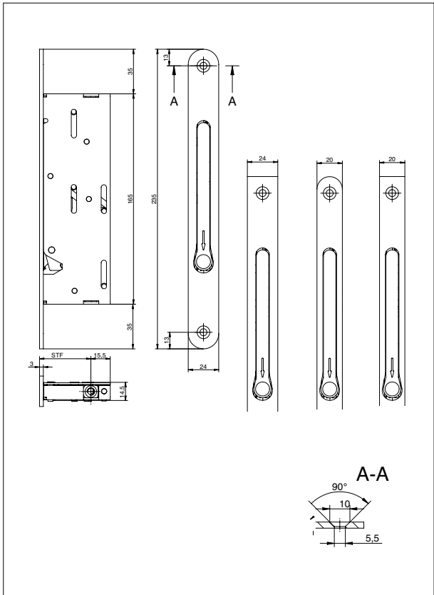
尺寸：GBS 94f 企口门插销锁
