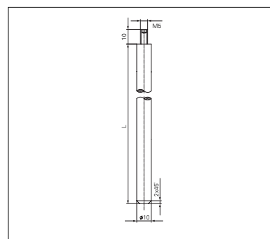
尺寸：门扇下置式联动销杆
