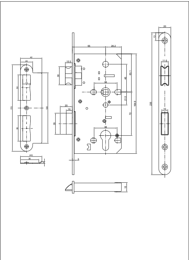
尺寸图: GBS 31 F NR 静音锁
