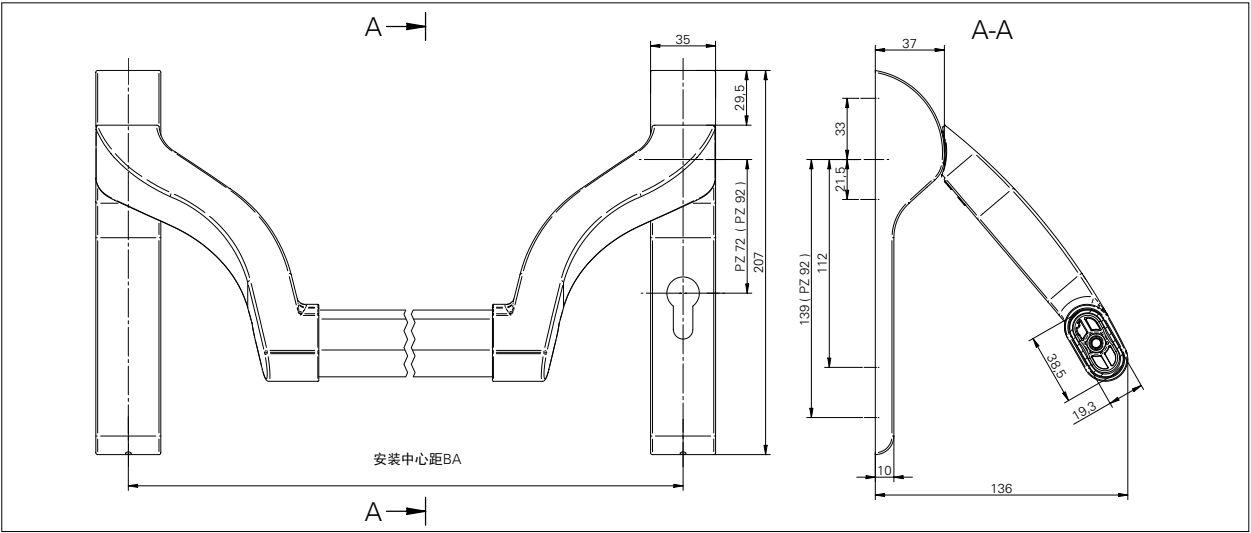
尺寸：EPN 900 IV
