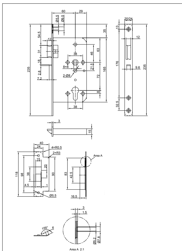
尺寸图: GBS 31 F NL夜锁
