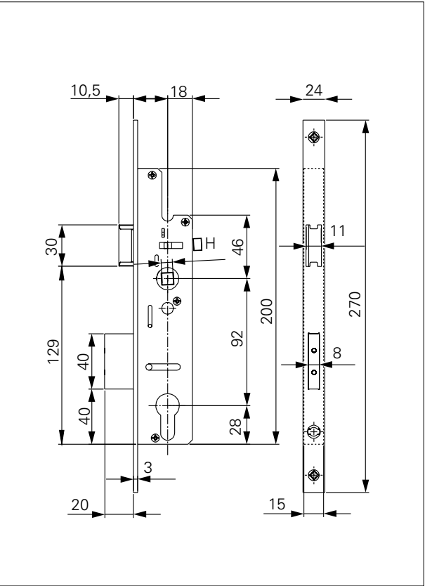
尺寸：GBS 60 型材门插芯锁
