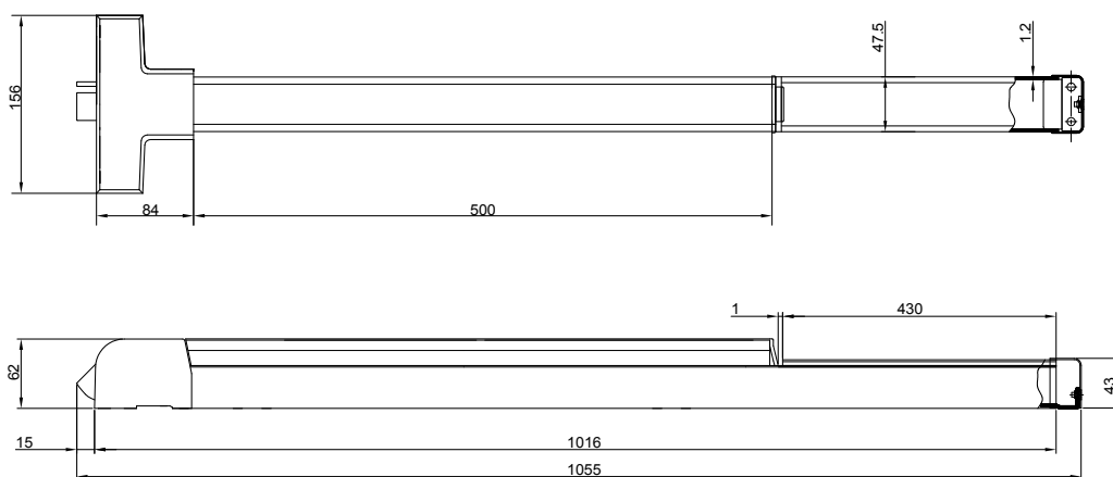
EPN 3000 单扇门锁紧
