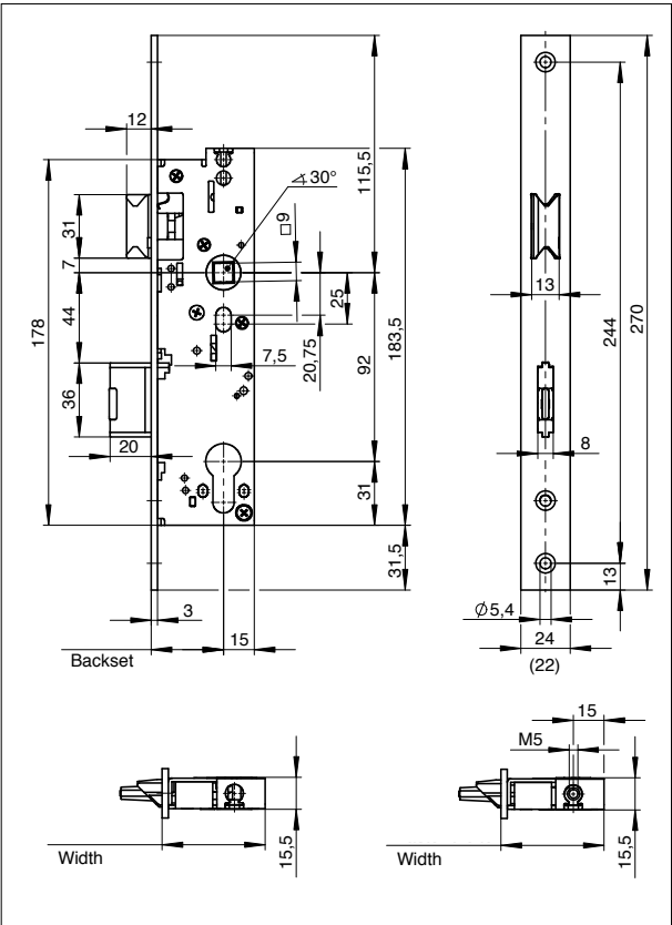
尺寸：GBS 97 双开型材门常开扇防火逃生门插芯锁
