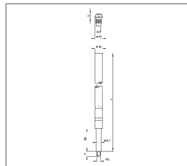
尺寸：门扇上置式联动销杆
