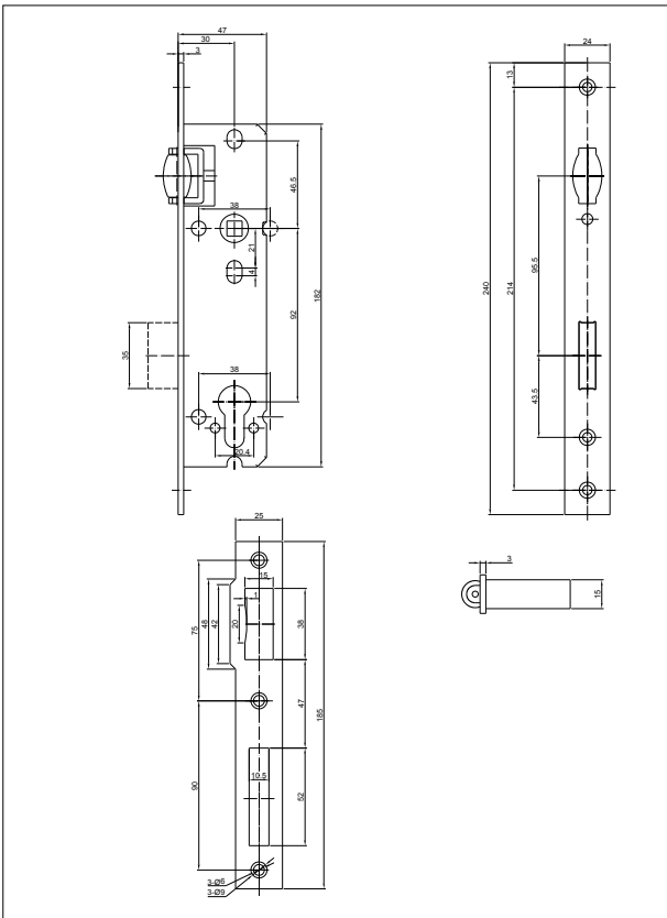
尺寸: GBS 31 F 窄体碰珠锁
