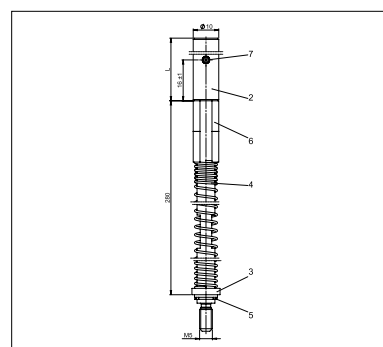
尺寸：门扇上置式联动销杆 GBS130/140
