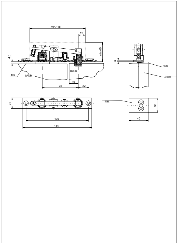
尺寸：碰珠斜舌型叠式锁系统 1
