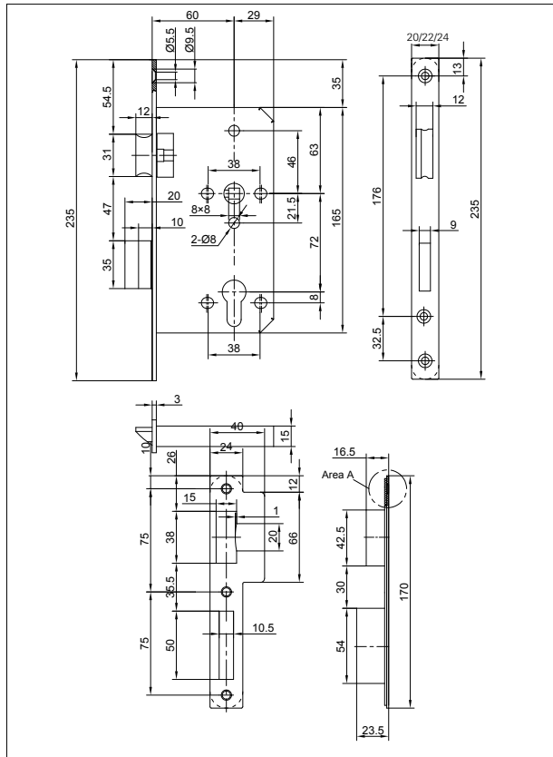
尺寸图: GBS 31 F SH 钢木门标准锁
