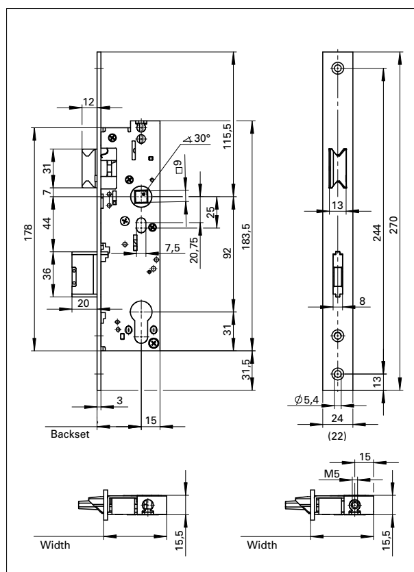
尺寸: GBS 96 型材门防火逃生门插芯锁
