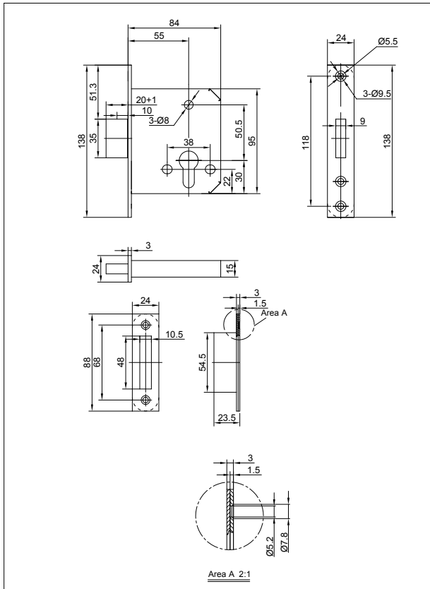
尺寸图: GBS 31 F SDB 单方舌锁
