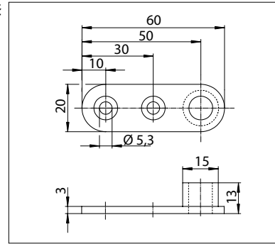
尺寸：联动式销杆门扇下置式导向套
