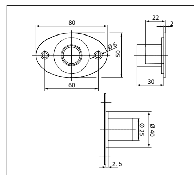
尺寸：地装式锁扣帽
