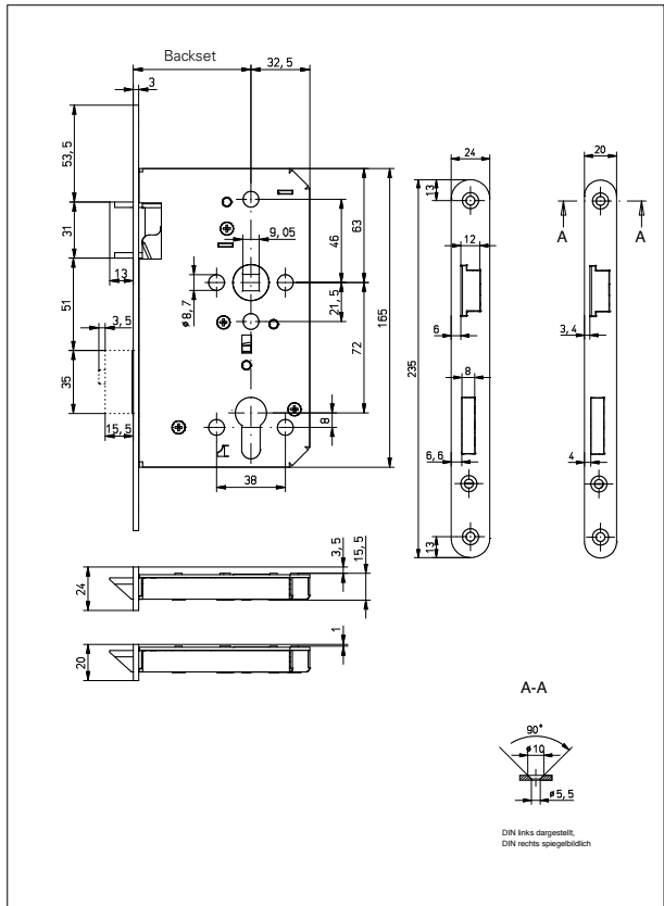
尺寸：GBS 93 双开门常开扇防火逃生插芯锁
