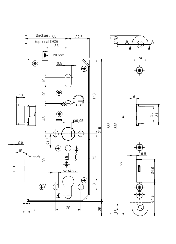
尺寸：GBS 140 防火插芯锁
