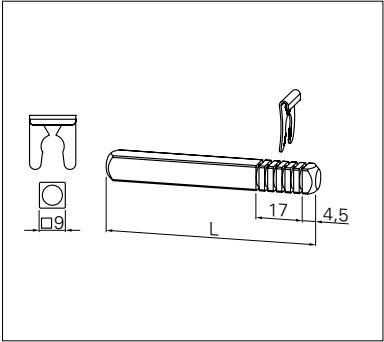
尺寸：半边卡片四方棒
