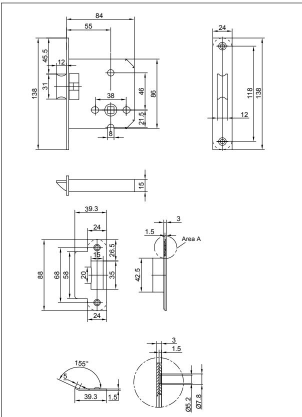
尺寸图: GBS 31 F SUR 单锋舌锁
