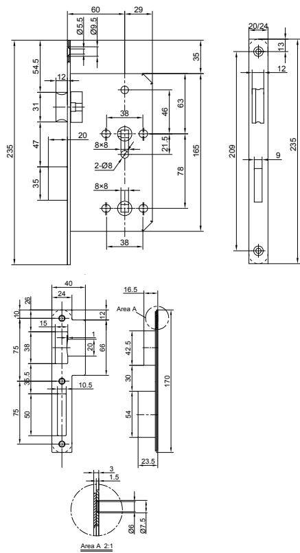
尺寸图: GBS 31 F WC浴室锁
