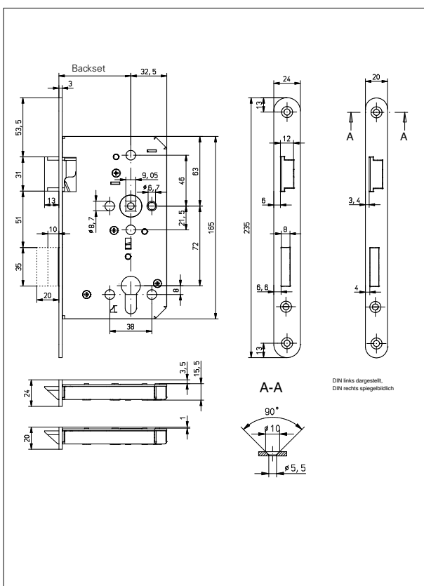
尺寸: GBS 92 防火逃生插芯锁
