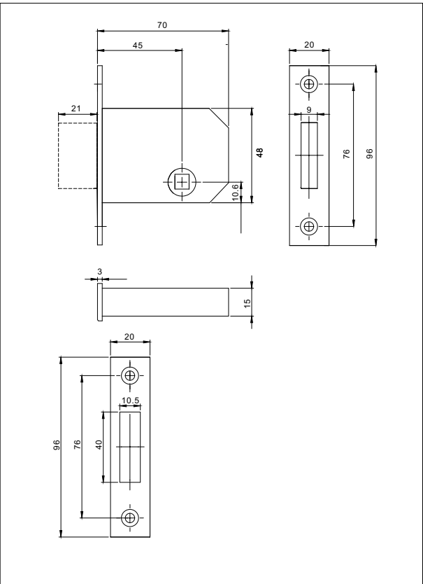
尺寸图: GBS 31 F SWC 卫浴单方舌锁
