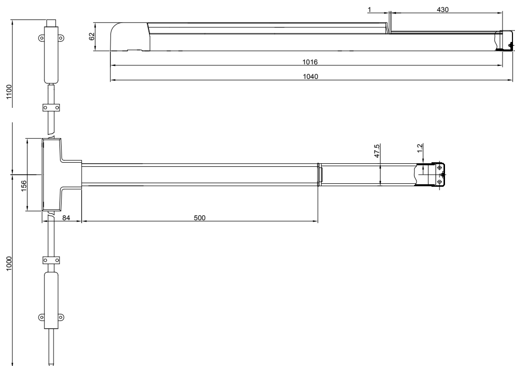
EPN 3000 适用于钢制/木质门单扇门，上下二点锁紧。
