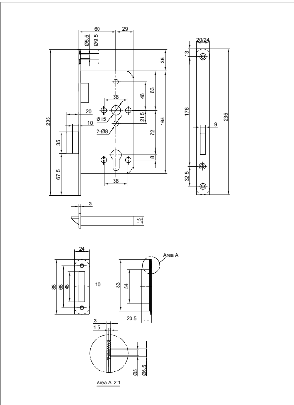
尺寸图: GBS 31 F DB 方舌锁
