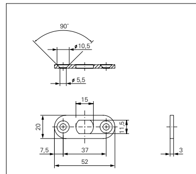
尺寸：门框下边沿锁挡片
