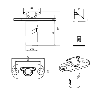
尺寸：门扇上置式调整锁
