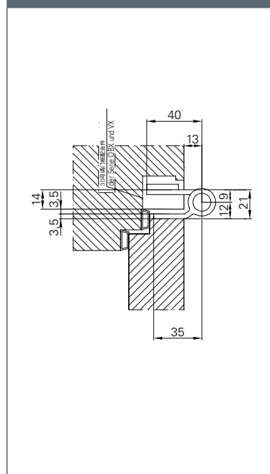
俯视图
