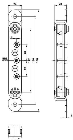
产品尺寸图
