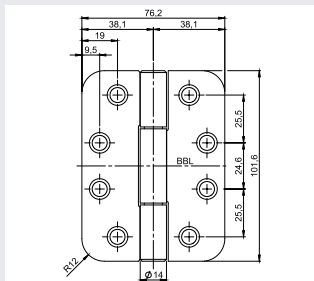
OBN-14 4030 C 圆角
