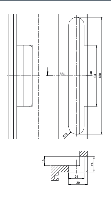
带装饰外盖铣切图
