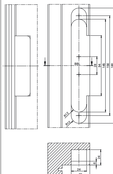
带装饰外盖铣切图
