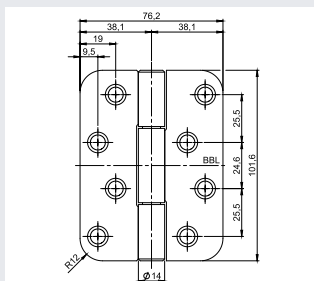
OBN-14 4030 Z 圆角
