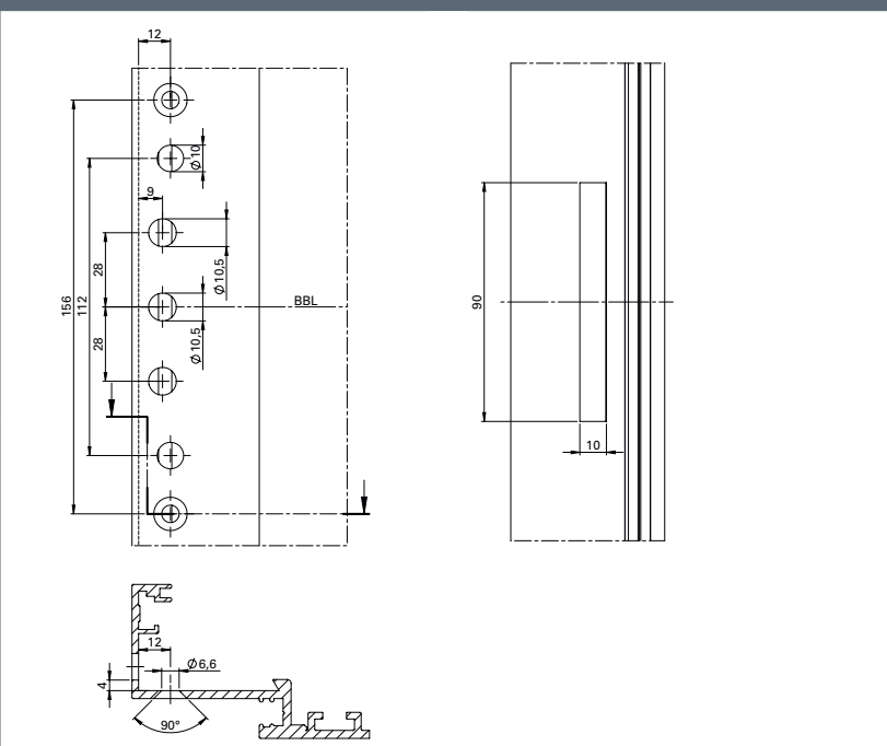
开孔尺寸图
