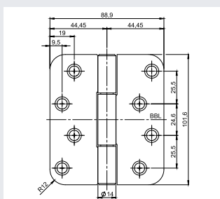
OBN-14 4035 Z 圆角
