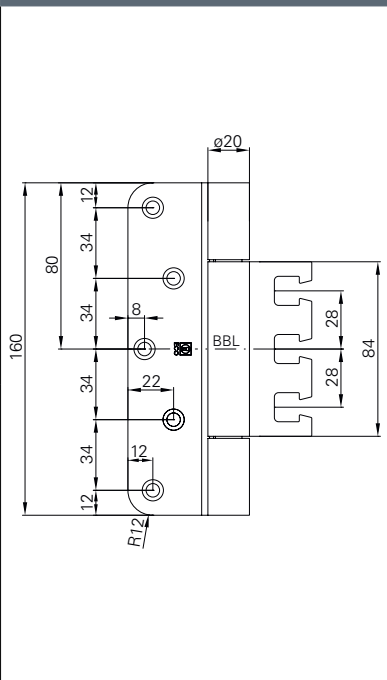
产品尺寸图
