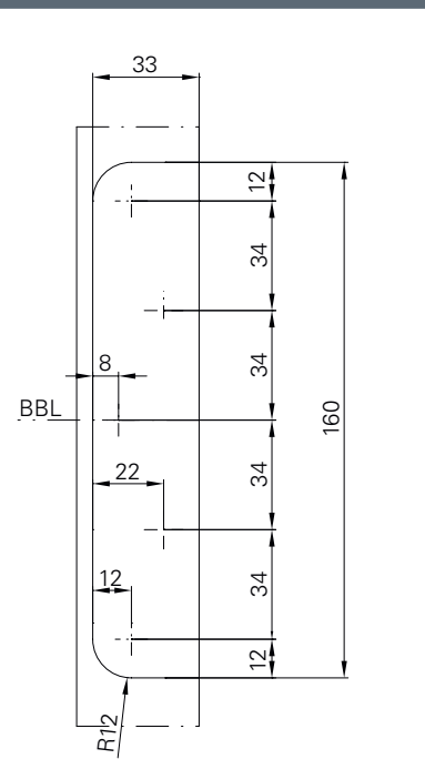
铣切图示
