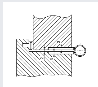
安装示意图
