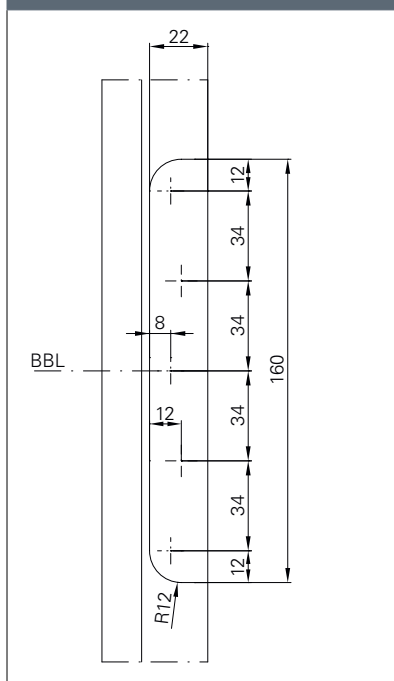
铣切图示
