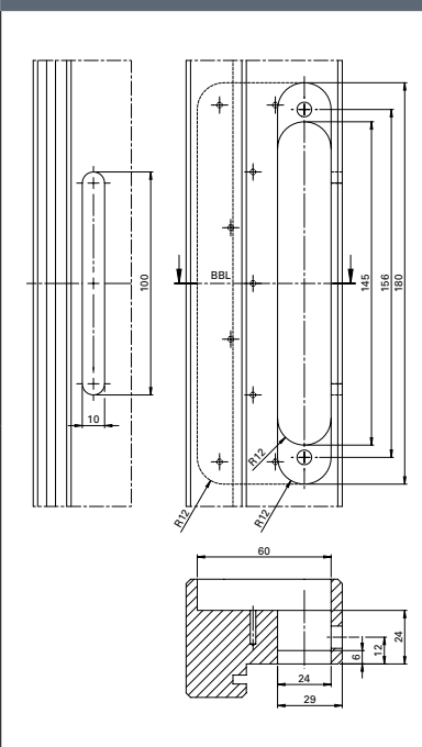
常规铣切图
