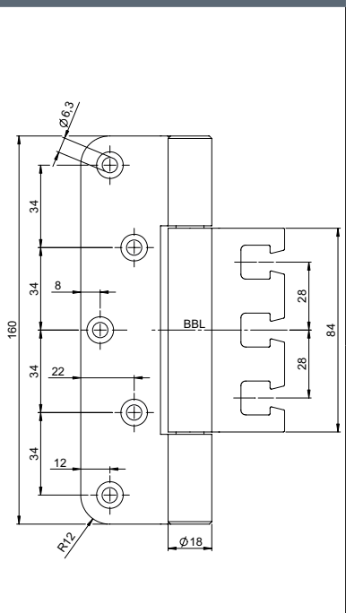
产品尺寸图
