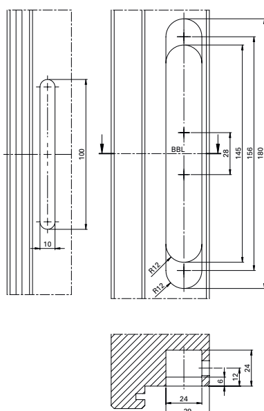
常规铣切图
