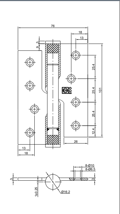
产品尺寸右手门图:
