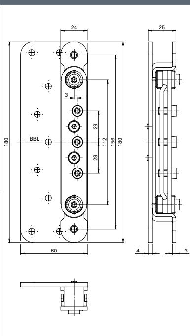
产品尺寸图
