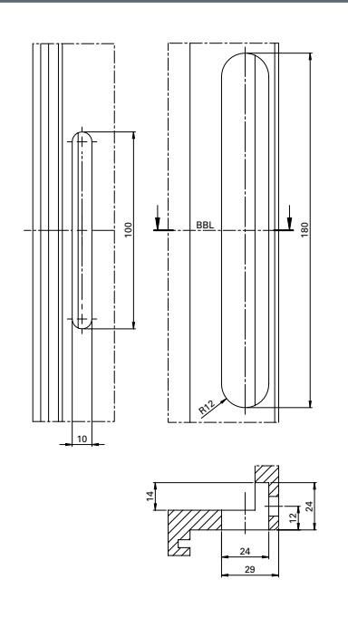
常规铣切图
