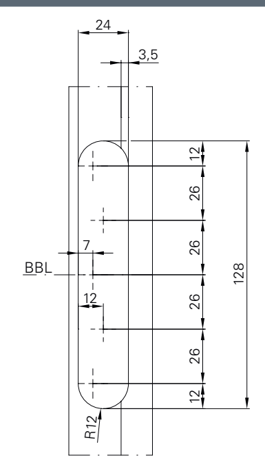
铣切图示
